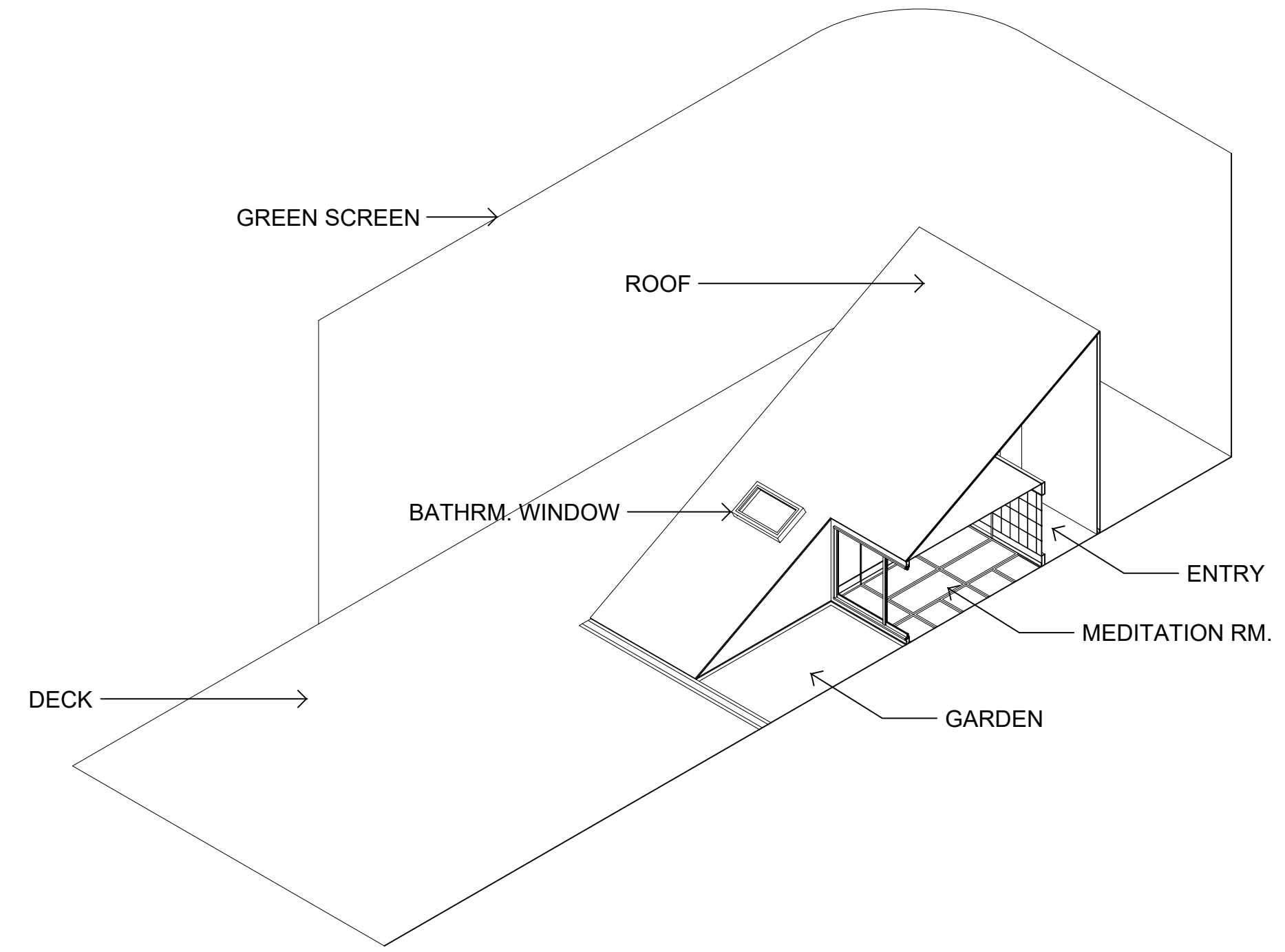
ISO SECTION ISO - NW CL-9 SCALE: 1/32" = 1'-0"
