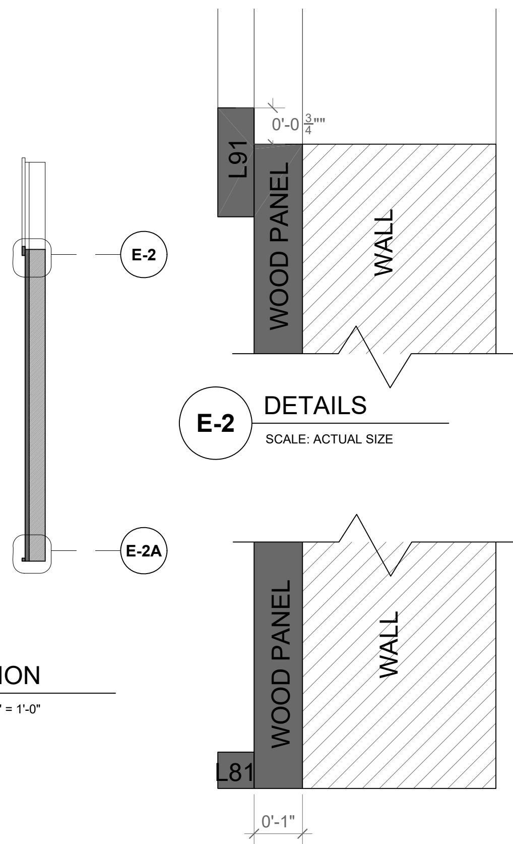
E-2A DETAILS SCALE: ACTUAL SIZE
