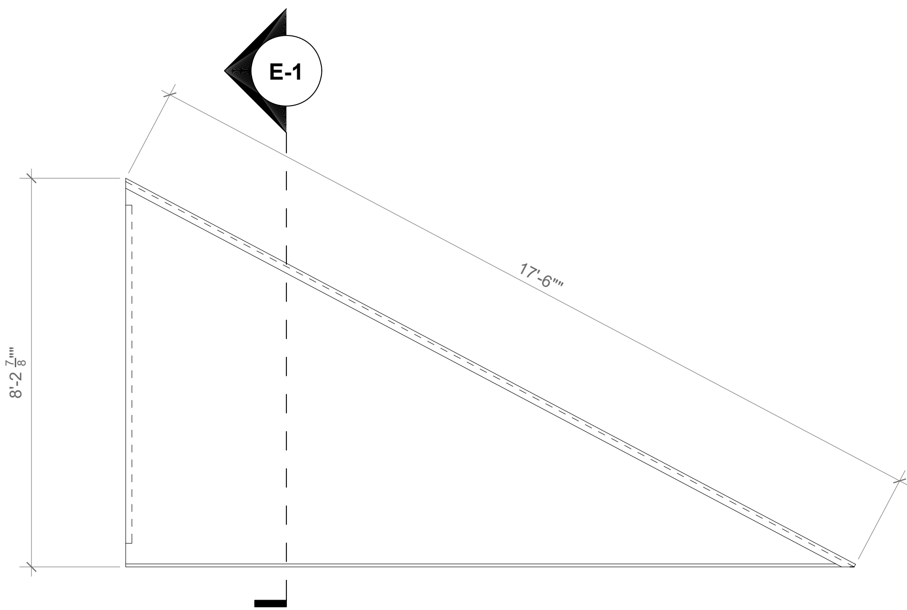
E ELEVATION, EXTERIOR WALL E SCALE: 1/2" = 1'-0"
