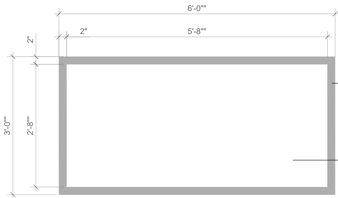
DT-1 TATAMI MAT DETAIL CL-7 SCALE: 1" = 1'-0"
